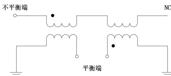
YLBL-40-E6-D产品原理图
